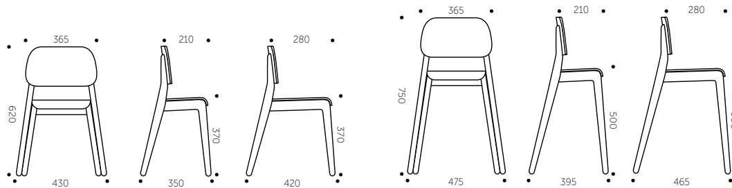
GROW-LASTENTUOLI IK 37 CM Istuinsyvyys 21 cm jalkatuella Tuotenro: 146618 Lisävaruste: Turvakaari Istuinsyvyys 28 cm Tuotenro: 146630 Lisävaruste: Jalkatuki
